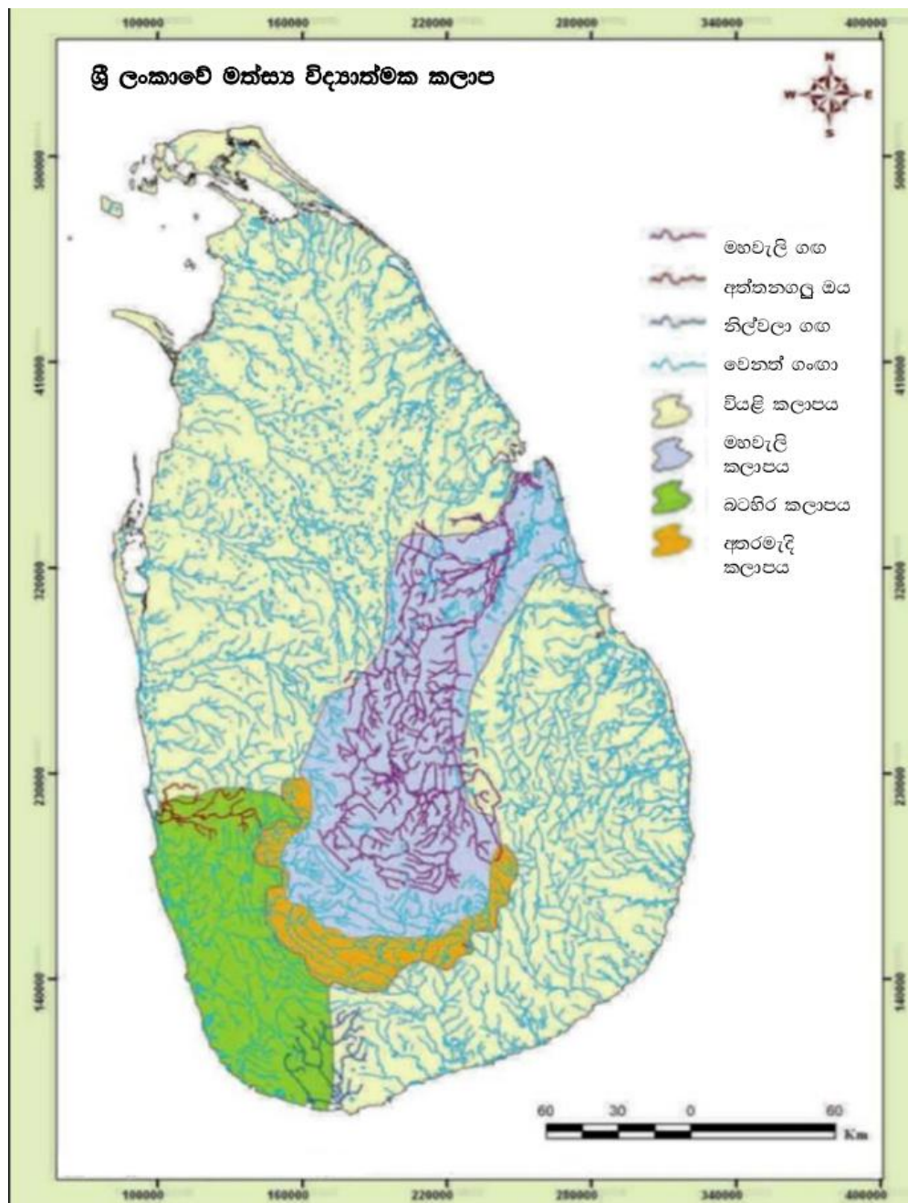
සිතියම් අංක 2: ශ්‍රී ලංකාවේ මත්ස්‍ය විද්‍යාත්මක කලාප
