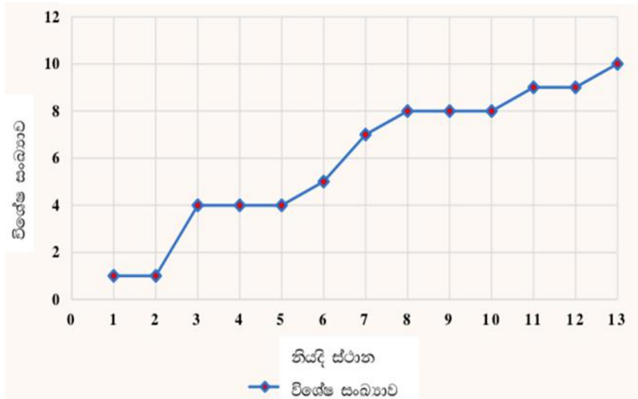
රූපසටහන් අංක 2: බලවතාව ඔයෙහි නියැදි ස්ථාන 13 ආශ්‍රිත මිරිදිය මත්ස්‍ය විශේෂවල සමුච්චිත සංඛ්‍යාත වක්‍රය
